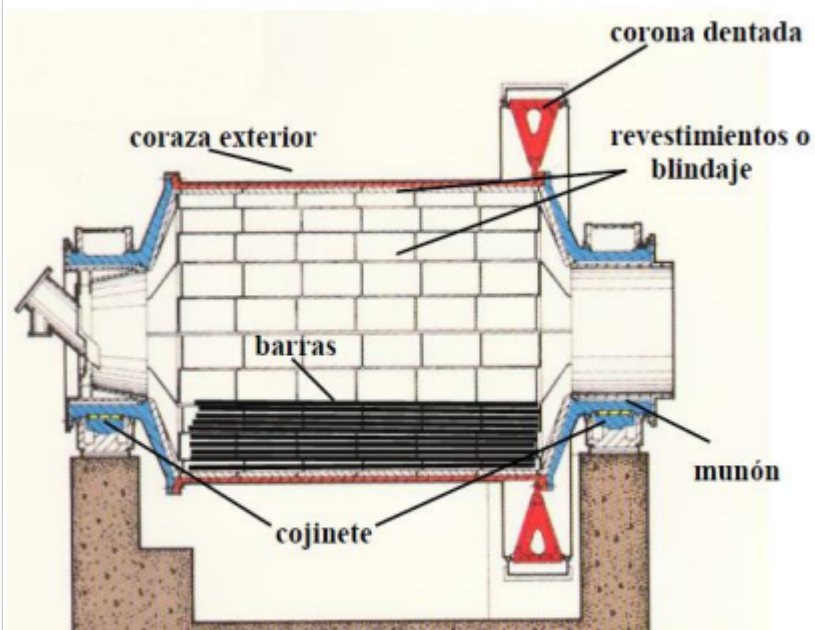
Figura 3. Molino de barras.
