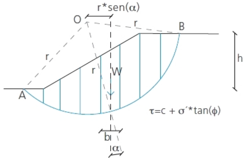
Figura 2. Esquema del análisis de estabilidad de taludes por el método de Fellenius
