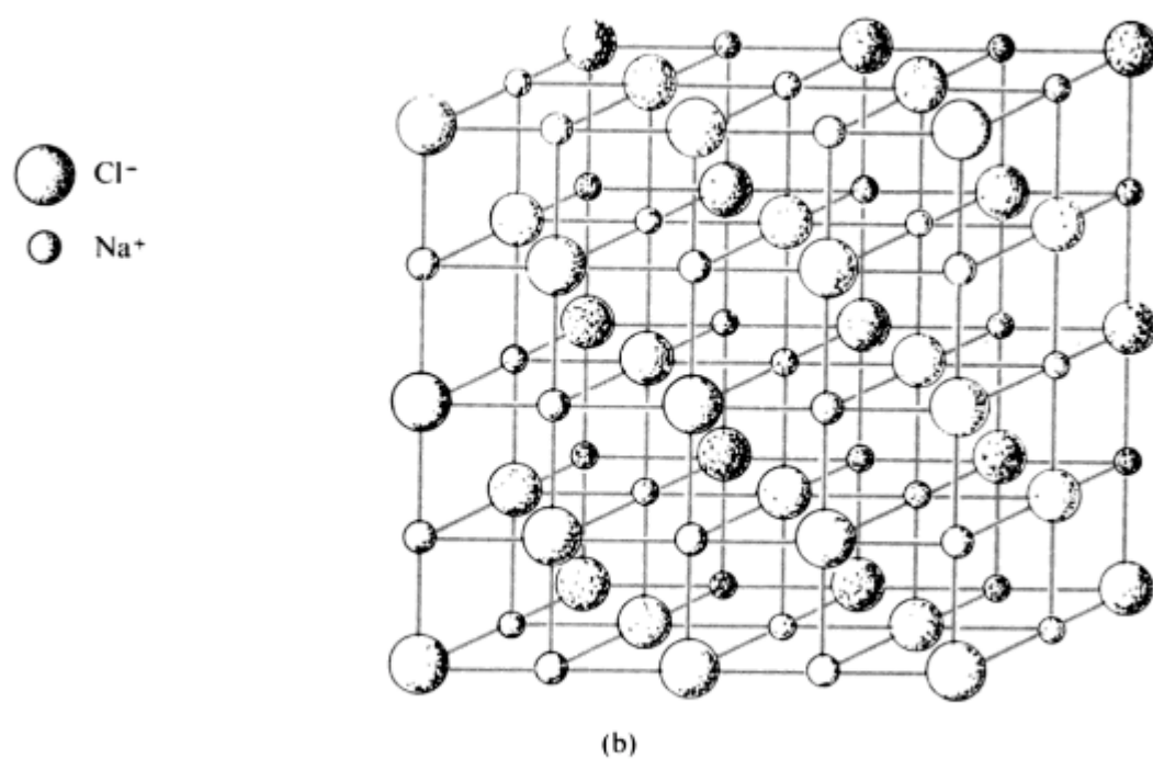
FIG. 1-1 (b) Modelo mostrando la ordenación geométrica de la estructura del cloruro sódico.
