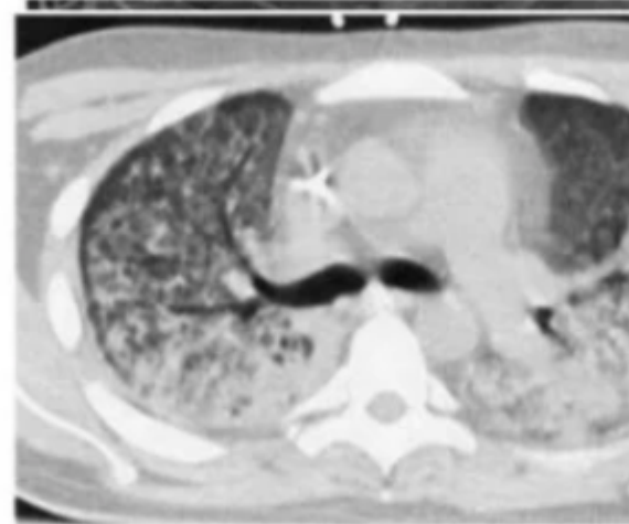
FIGURA 262-4. Tomografía computarizada representativa durante la fase exudativa del ARDS, en la cual predominan las opacidades alveolares en zonas de base y la atelectasia. (Inglaterra).
